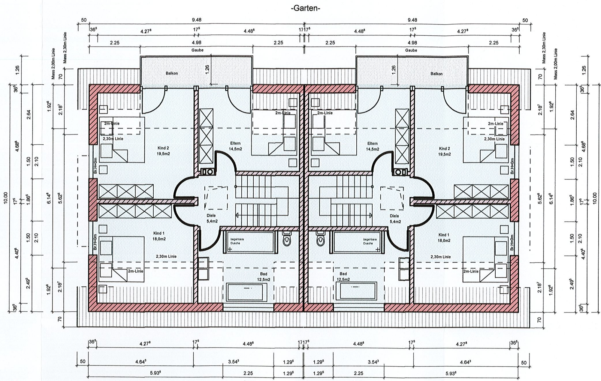
Grundriss OG
