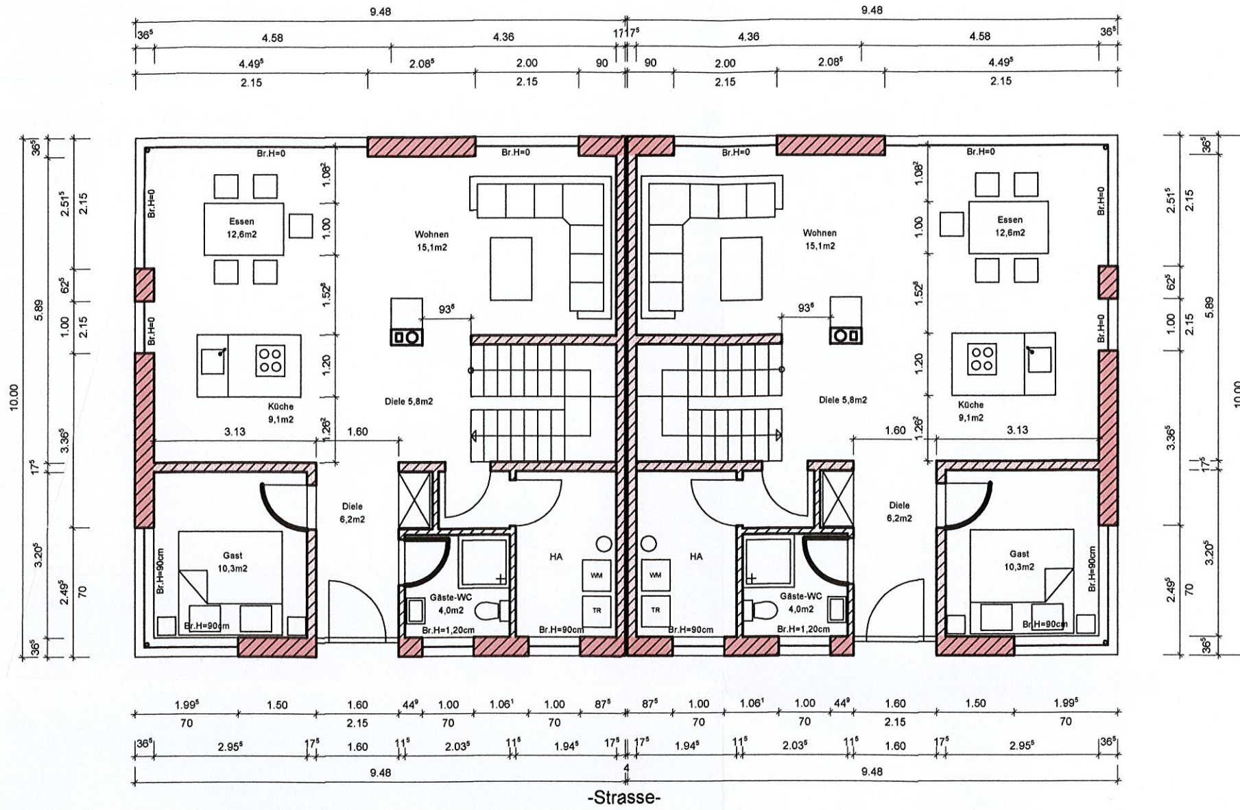
Grundriss EG
